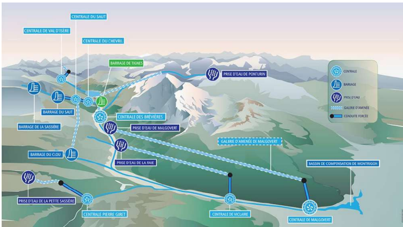
Schéma de l'aménagement hydroélectrique de Tignes-Malgovert
